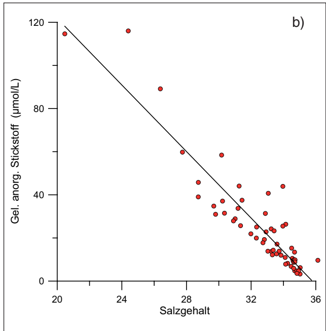
Abb. 3: Korrelation zwischen Phosphat und Salzgehalt (a) und gelöstem anorganischen Stickstoff (DIN) und Salzgehalt (b) im Wattenmeer und in der Deutschen Bucht im Jahre 2006. Nur Oberflächenproben werden berücksichtigt
