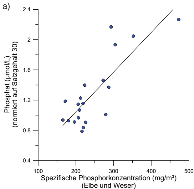
Abb. 5a: Korrelation zwischen den spezifischen Phosphorkonzentrationen der Elbe und Weser (Jahreseintrag/Jahresabfluss) und den auf Salzgehalt 30 normierten Konzentrationen des Phosphats in der Deutschen Bucht und im Wattenmeer ( R^2 = 0,68 ; p < 0,00001 ; n = 20 )
